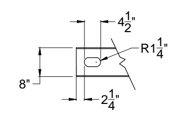
LUG DETAIL 'A'
