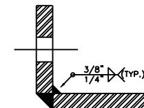
TYP FLANGES WELD DETAIL
