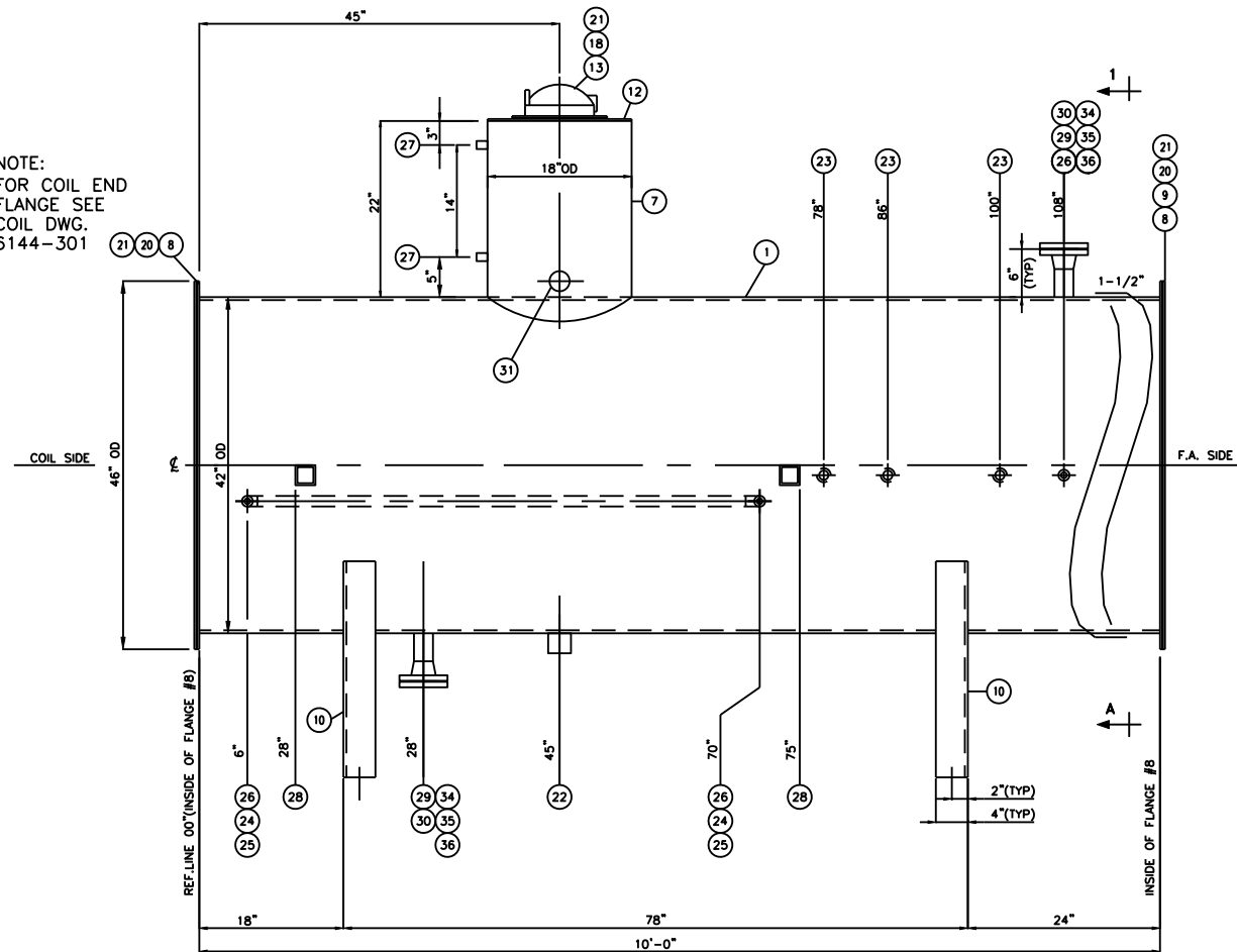
ELEVATION
