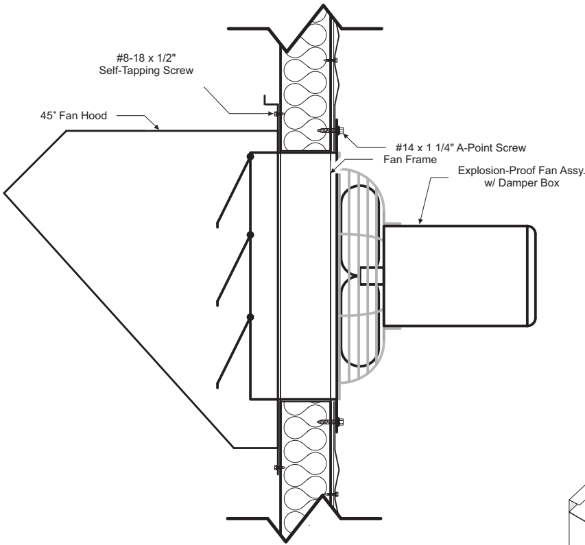
Fan Detail (TYP)
