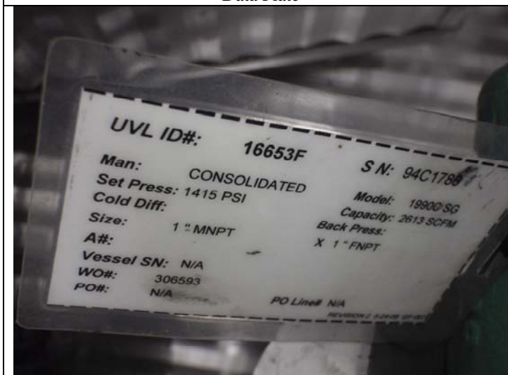
PSV Tag
